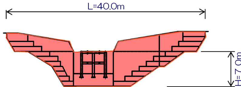
堰堤一般図
