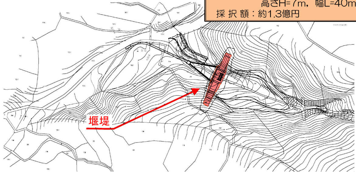
堰堤一般図
