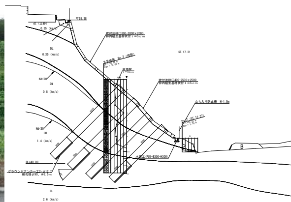
標準断面図
