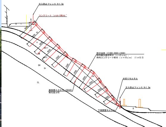
標準断面図
