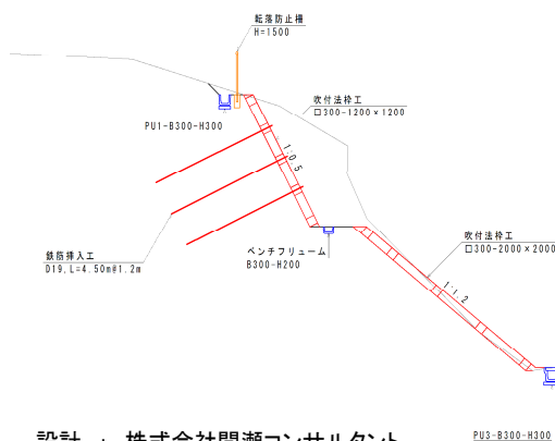
標準断面図
