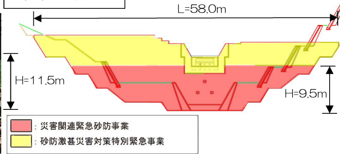
堰堤一般図
