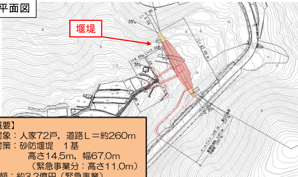
堰堤一般図
