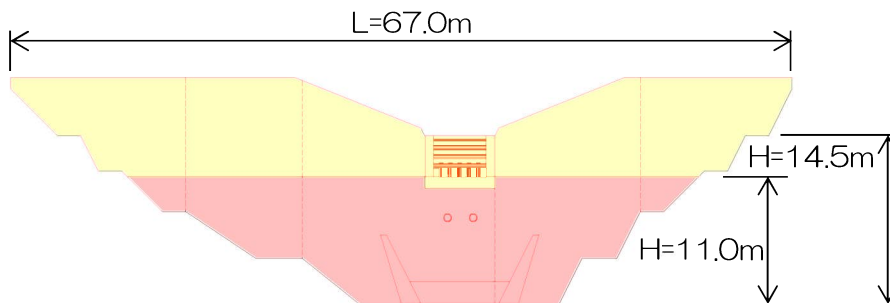
堰堤一般図
