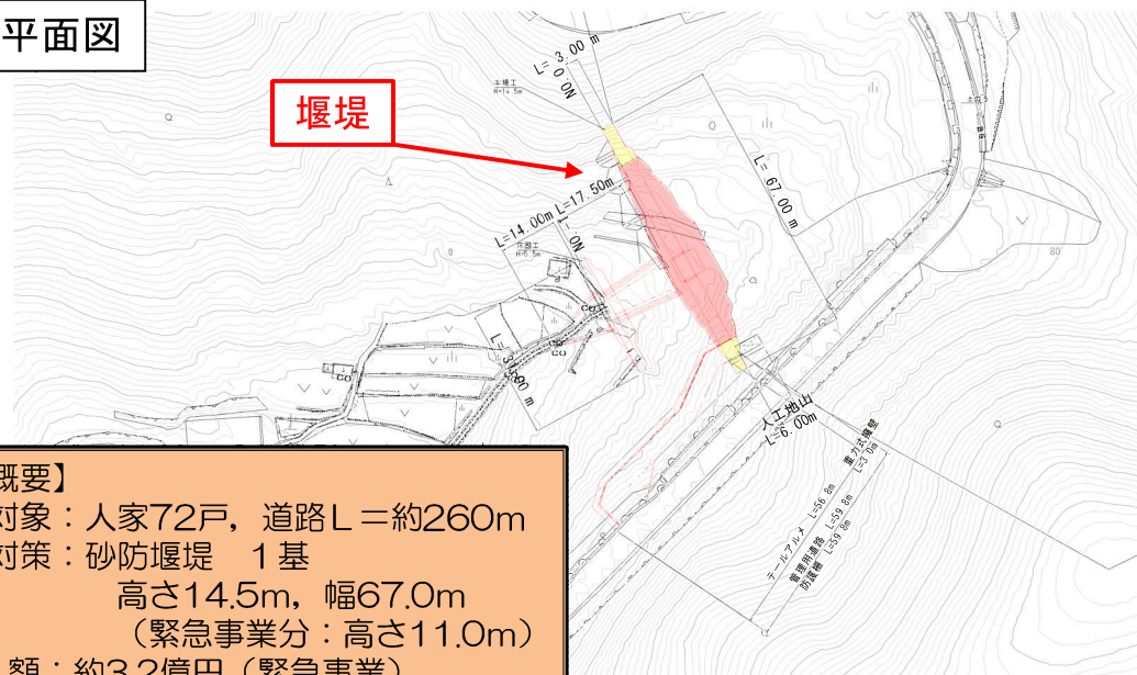
堰堤一般図
