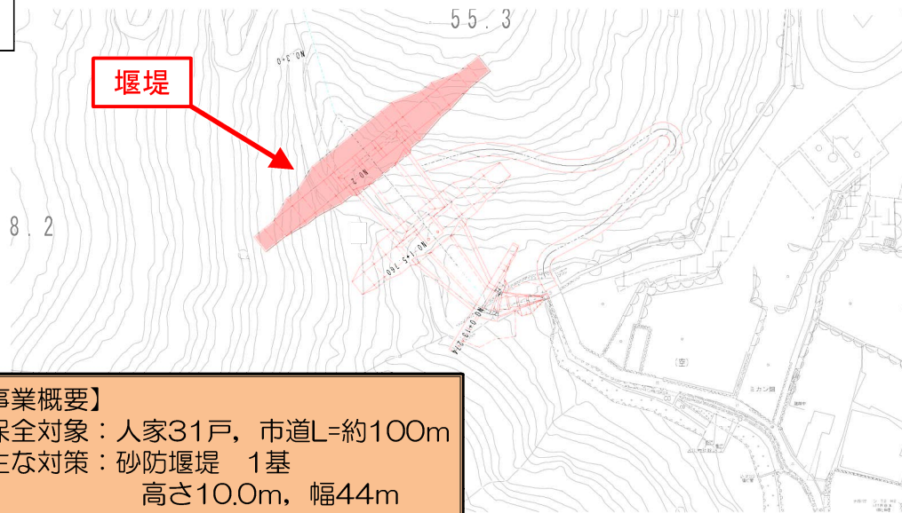
堰堤一般図
