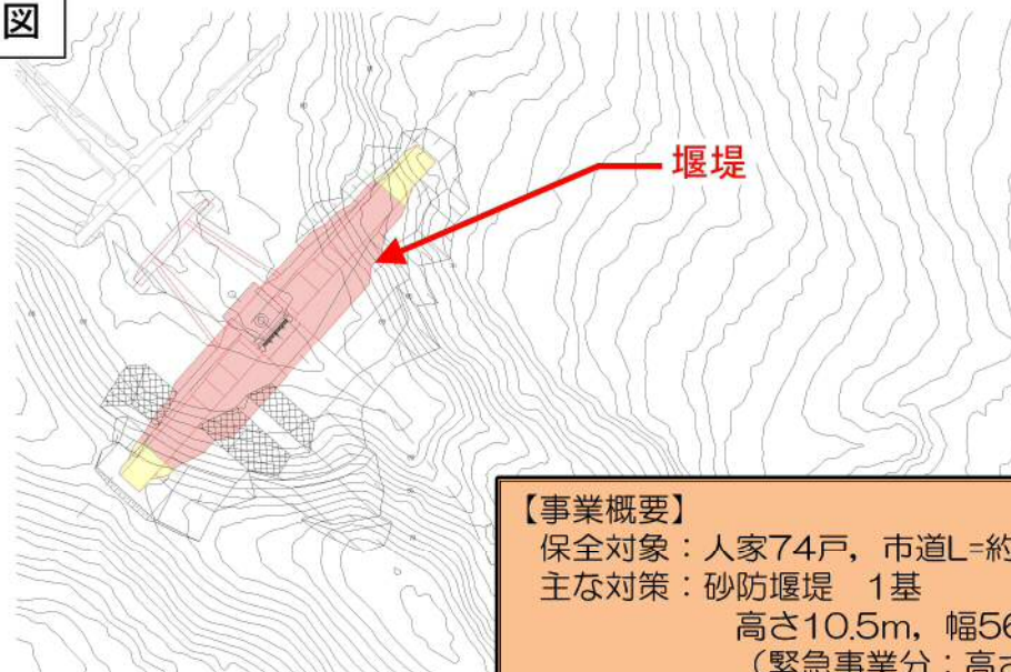
堰堤一般図
