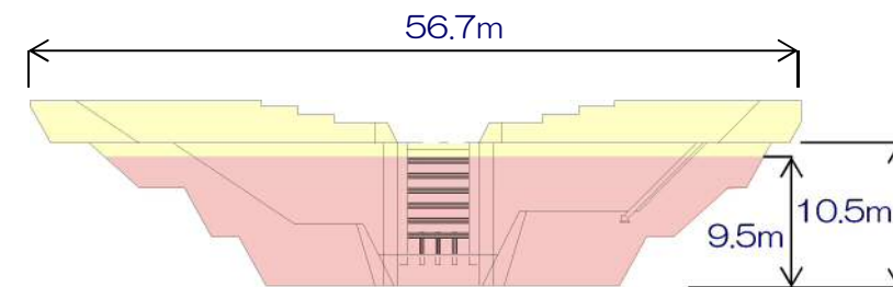
堰堤一般図
