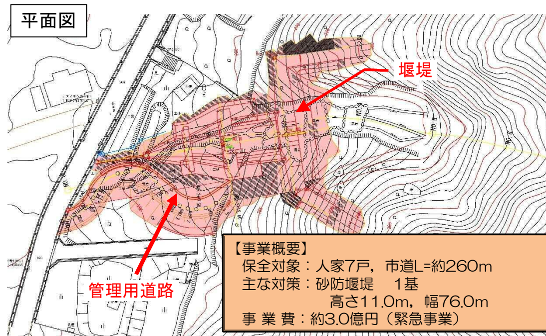
堰堤一般図
