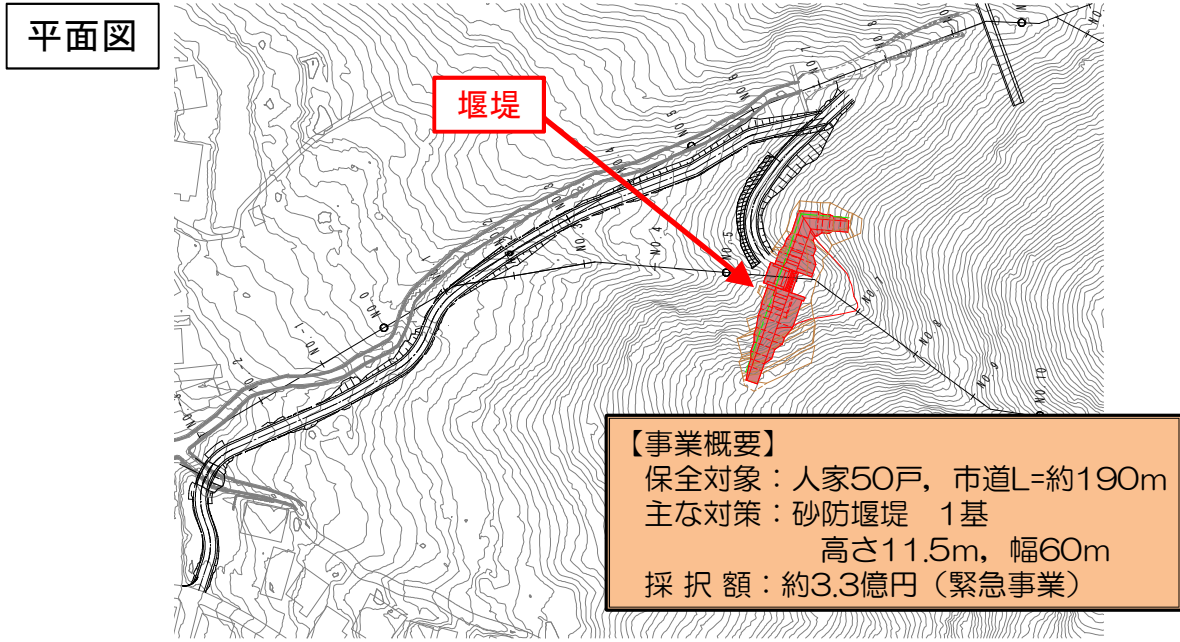
堰堤一般図
