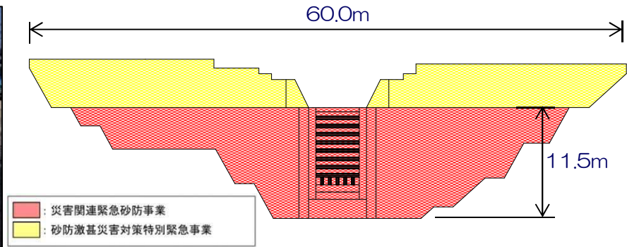
堰堤一般図
