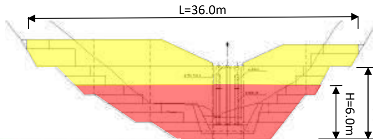
堰堤一般図
