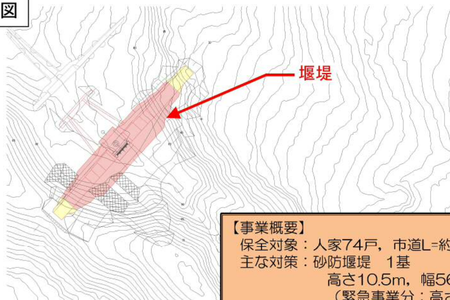
堰堤一般図
