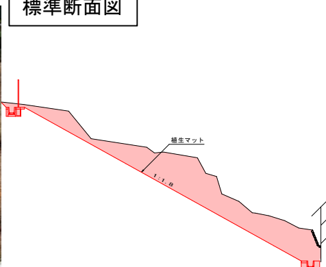
標準断面図
