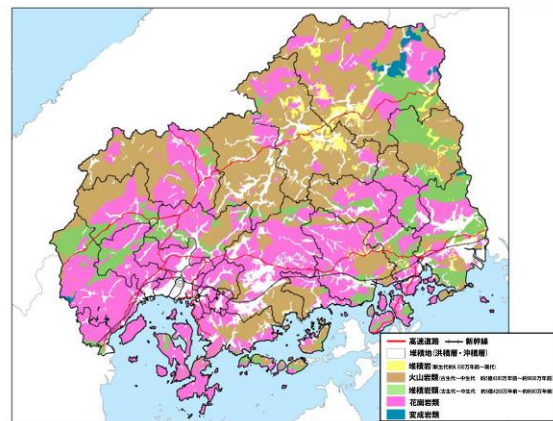
図 1.1.5 本県域の地質分布図
