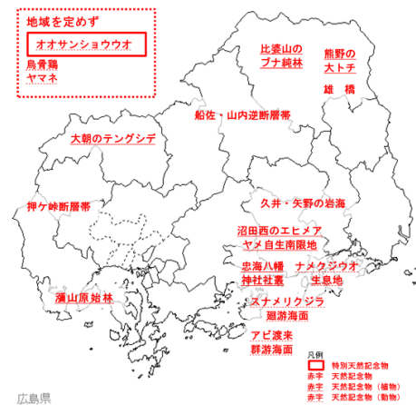
図 1.2.7 国指定天然記念物の分布*
