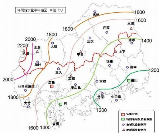
図 1.1.6 本県域の年間降水量平年値図
