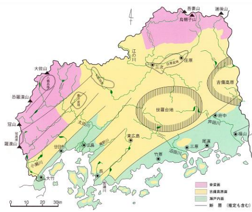
図 1.1.3 本県域の地形 (広島県立歴史民俗資料館作成図に加筆)
