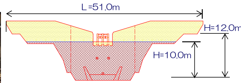
堰堤一般図
