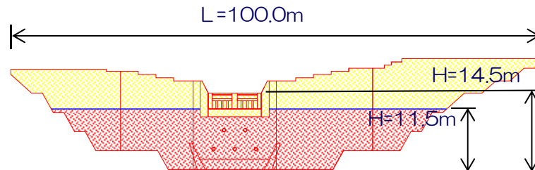
堰堤一般図
