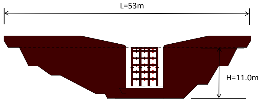
堰堤一般図
