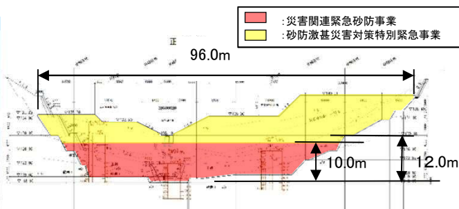
堰堤一般図
