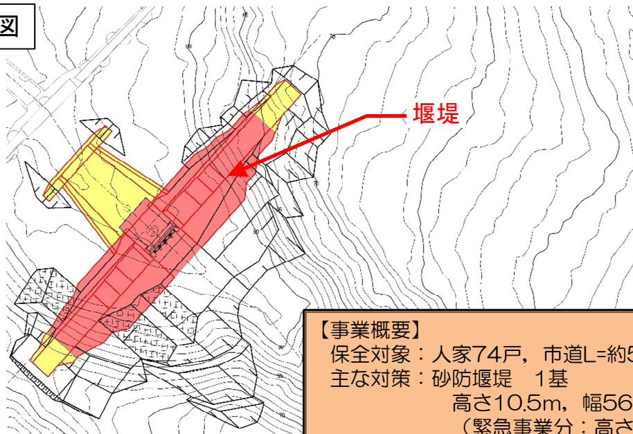
堰堤一般図
