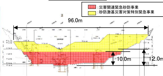
堰堤一般図
