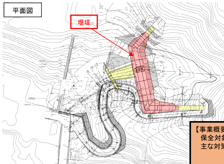
堰堤一般図
