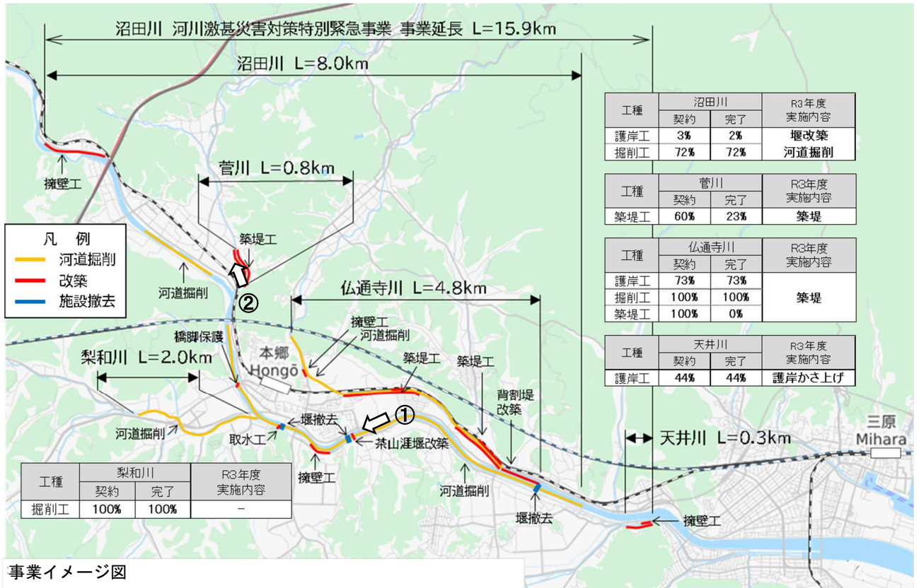
《沼田川【河川激甚災害対策特別緊急事業】の進捗状況》 【平面図】
