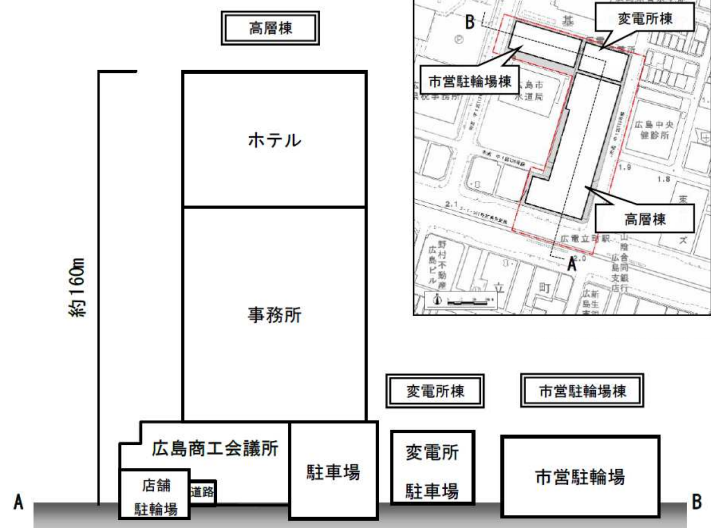
断面図
