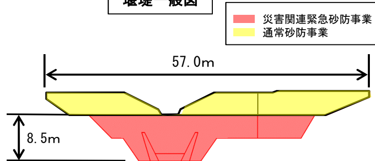
堰堤一般図
