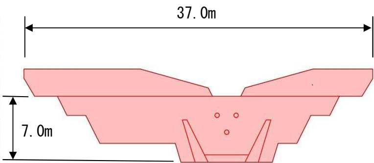
堰堤一般図
