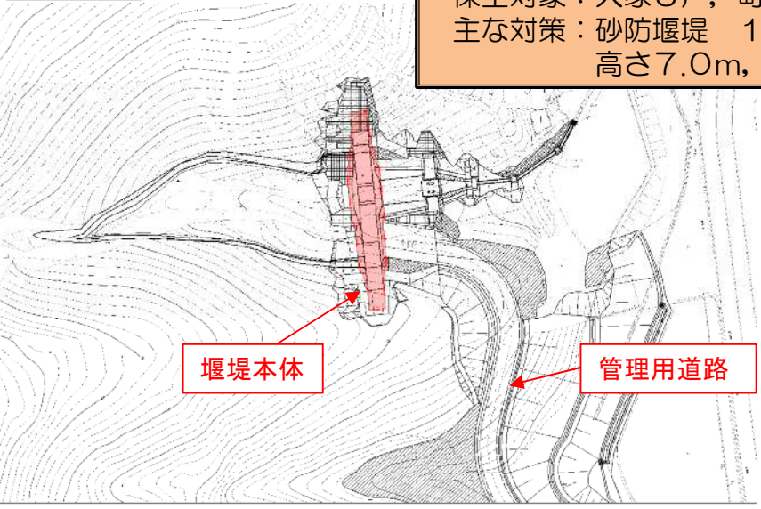
堰堤一般図
