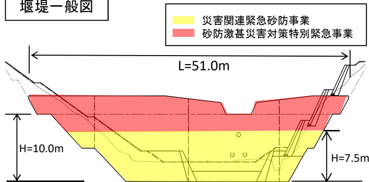
堰堤一般図
