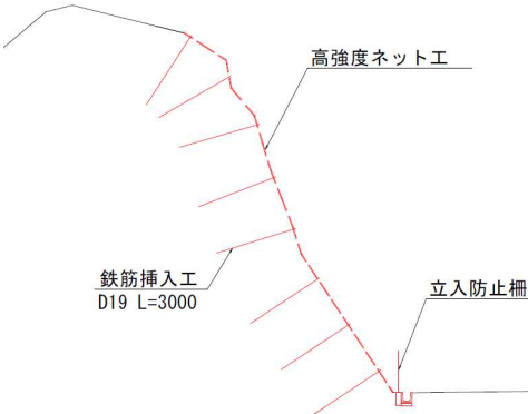
標準断面図
