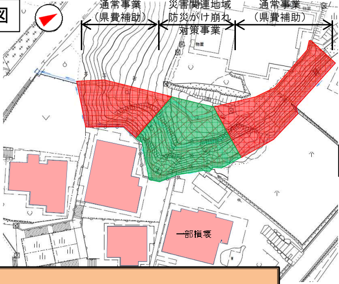
斜面崩壊・被災状況（H30年7月）
