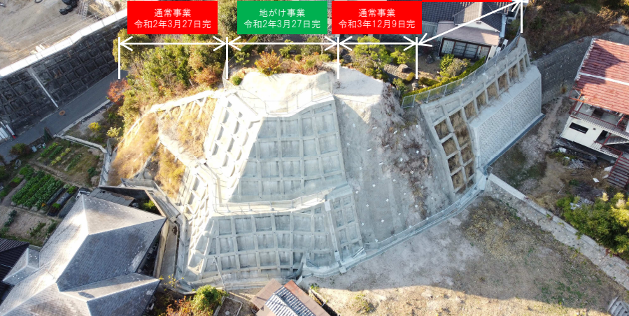
工事完了（令和3年12月9日）
