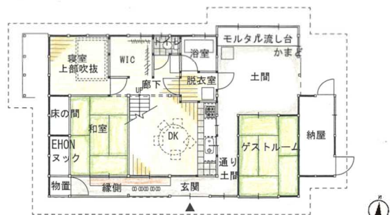
1階平面図 (リフォーム後)
