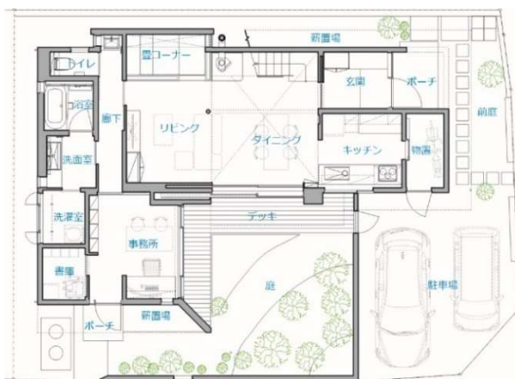
1 階平面図
