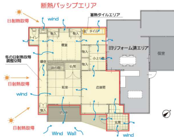
1階平面図 (リフォーム後)
