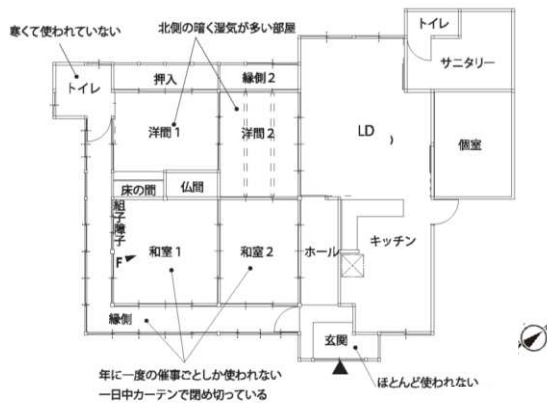
1階平面図 (リフォーム前)
