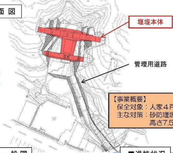
堰堤一般図
