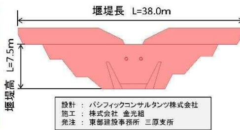
堰堤一般図
