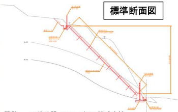
標準断面図
