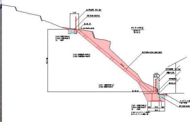
標準断面図
