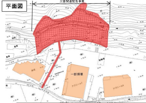
斜面崩壊・被災状況（令和2年7月14日）
