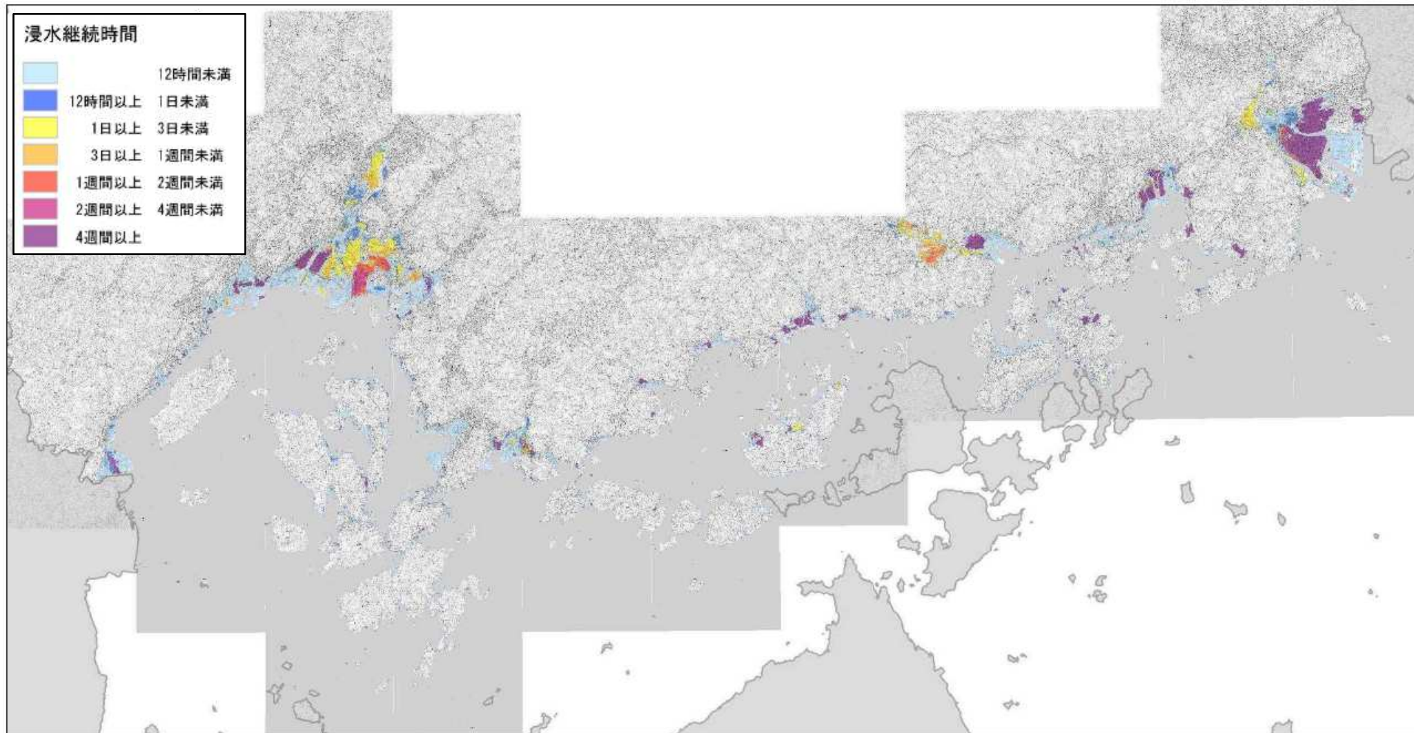
図1. 高潮浸水想定区域図（浸水継続時間）（広島県沿岸全域イメージ図）
