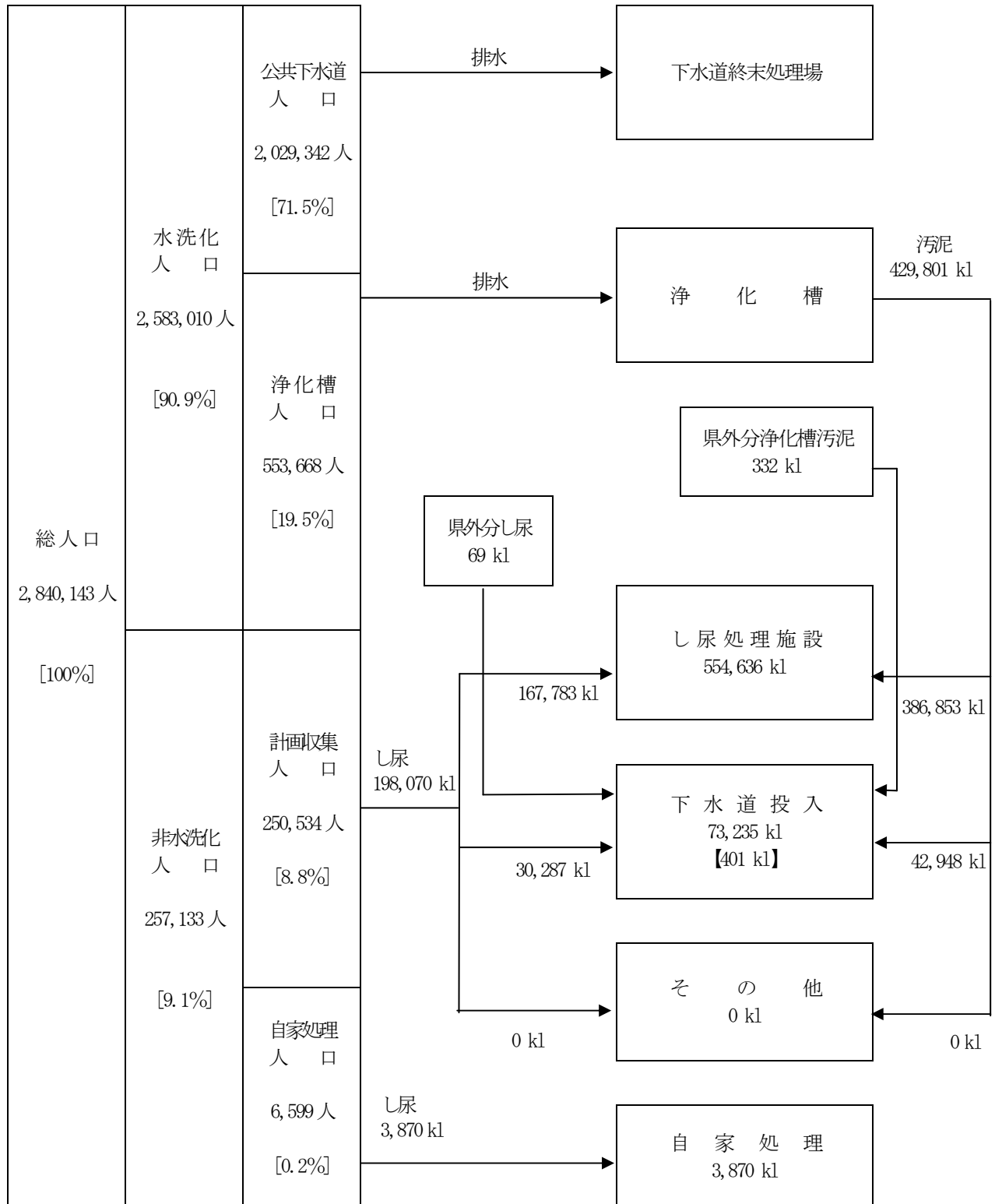
図 3 - 1 し尿処理及び浄化槽汚泥処理の概要（平成 30 年度）
