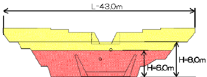
■ 堰堤一般図
