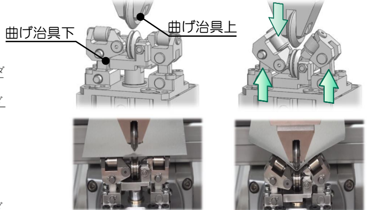
●曲げ治具の押し込み量 制御機構
