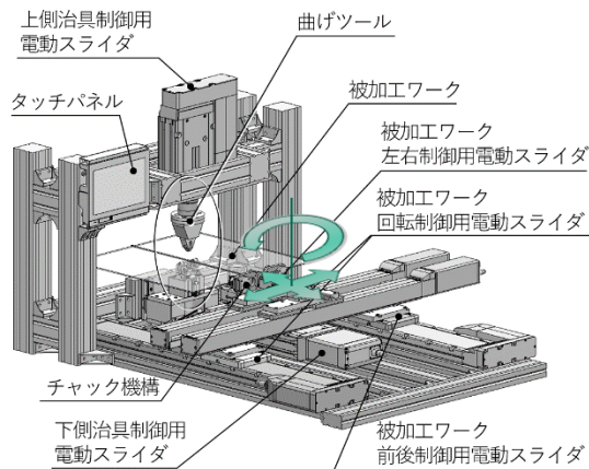
●薄板の位置・姿勢制御機構
