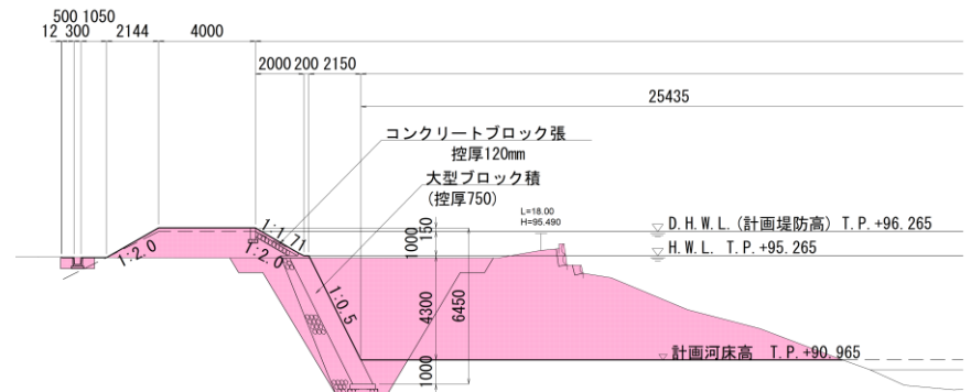
標準断面図 (A-A)
