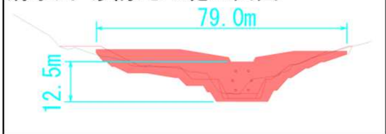
清水川 砂防えん堤正面図
