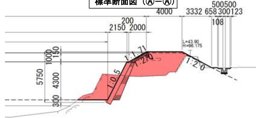
標準断面図 (A-A)
