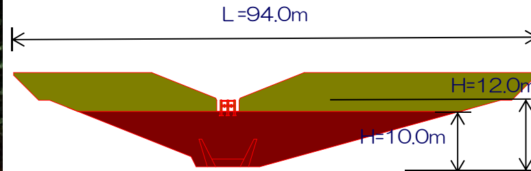
堰堤一般図
