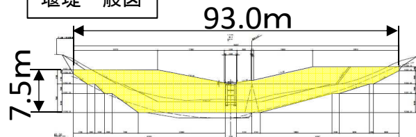
堰堤一般図
