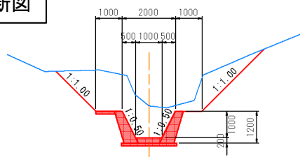
横断面図
