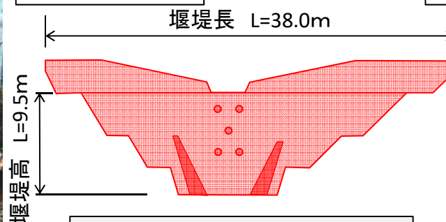
堰堤一般図
