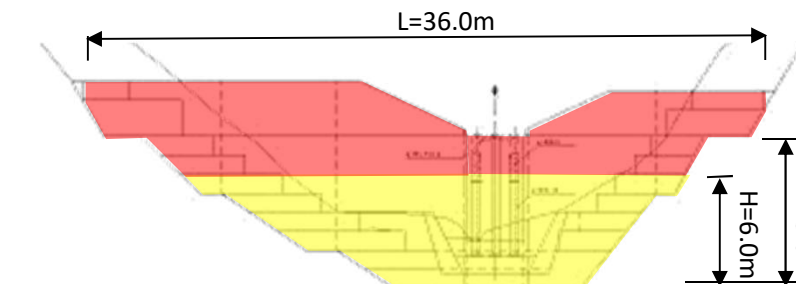
堰堤一般図
