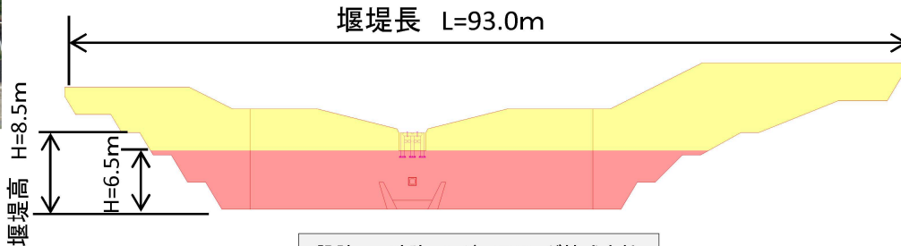
堰堤一般図
