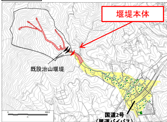
堰堤一般図
