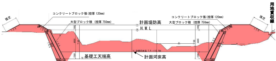
図2 河川改修イメージ
