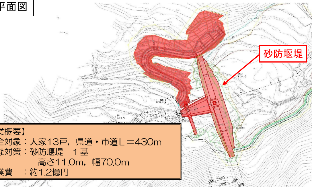
堰堤一般図
