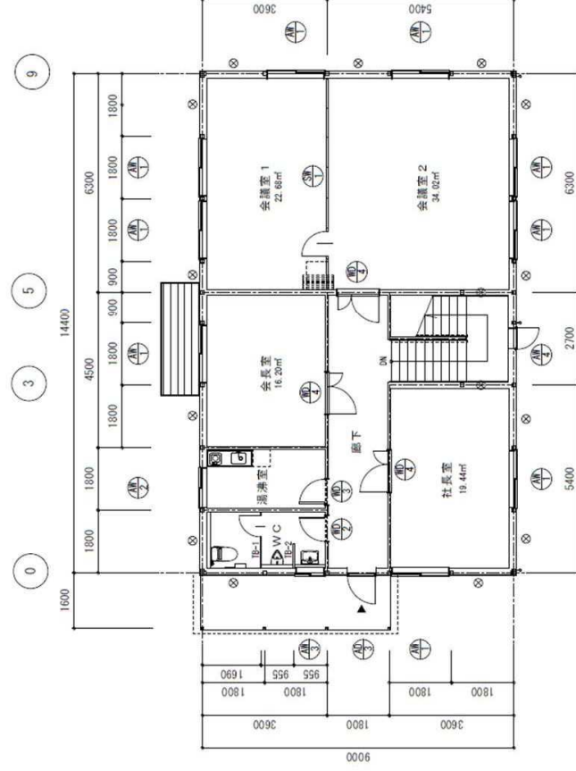
2階平面図
