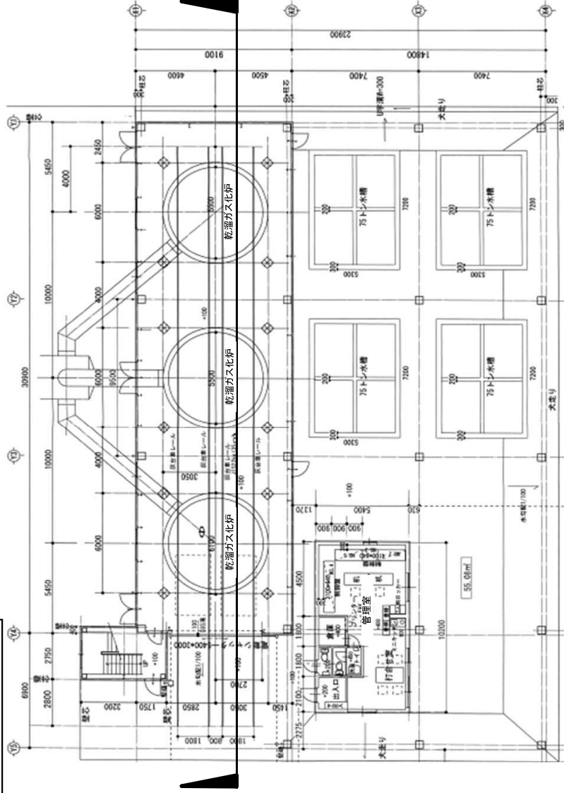
1 階 平 面 図
