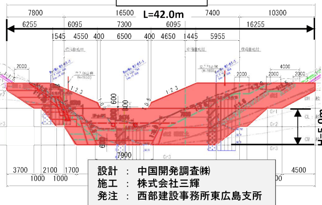
堰堤一般図
