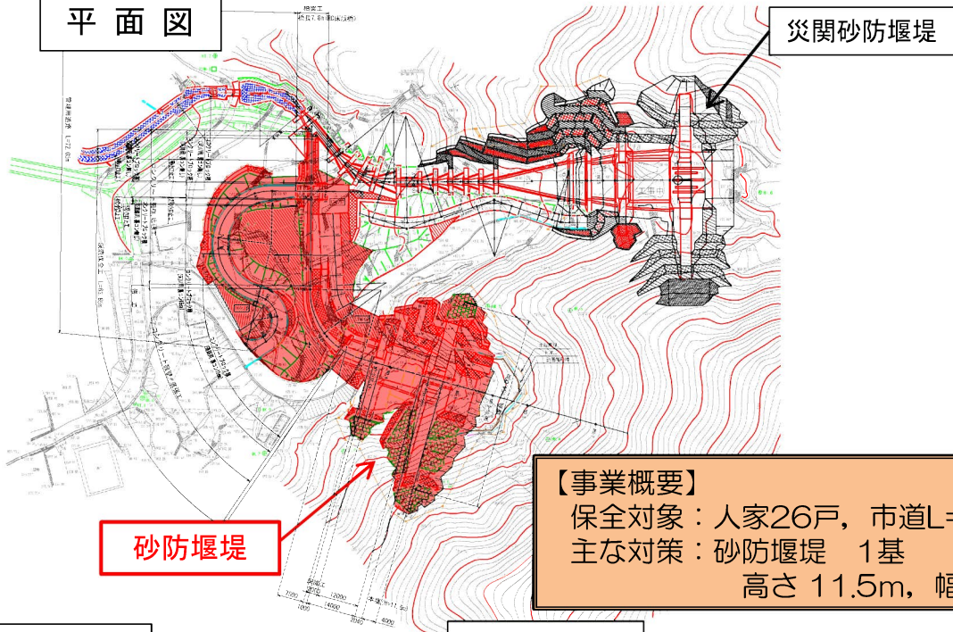
堰堤一般図
