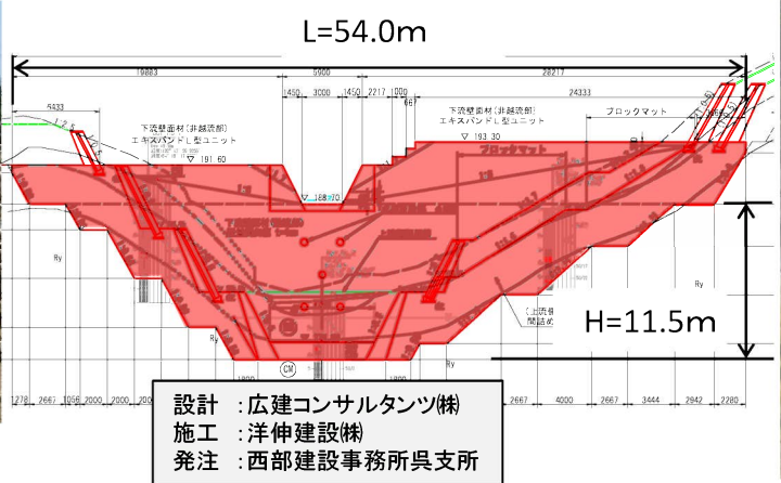
堰堤一般図
