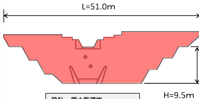
堰堤一般図
