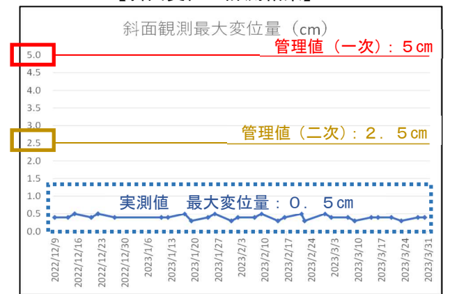
【斜面変位の計測結果】
